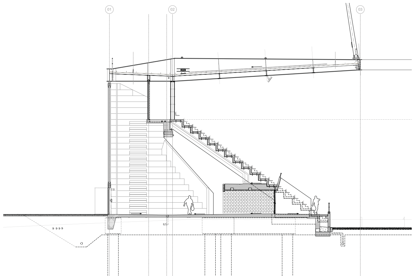
Coupe tribunes B-C-D
