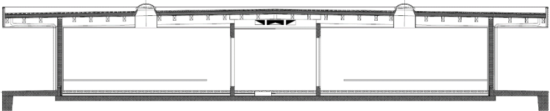
Coupe B / Schnitt B
